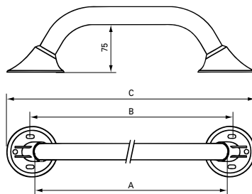
lengte A is de greepmaat
